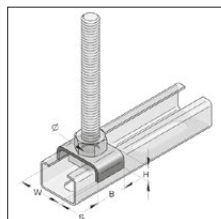
Podkładka profilowa
